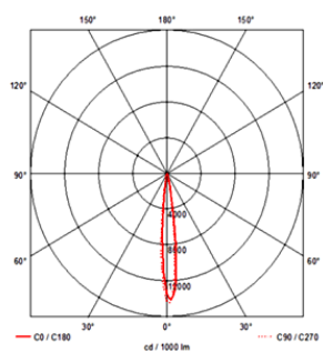
ADD0 75 T 12°
