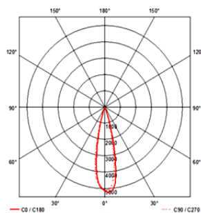
ADD0 75 T 24°
