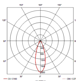
ADD0 75 T 36°
