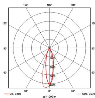
BONTEBOK 145 R 12°
