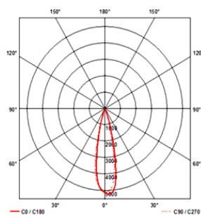
BONTEBOK 145 R 24°
