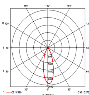
ETOSHA 130 R 38°
