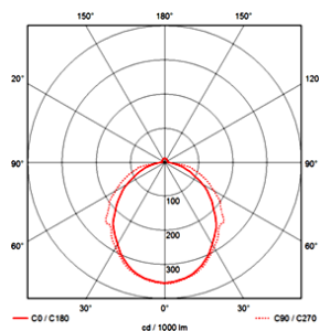
GARAMBA 120°
