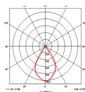
TULI 130 R - 60°
