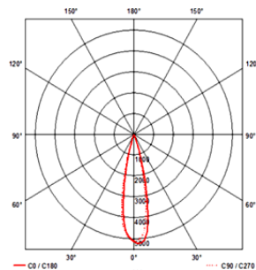
TULI 130 R - 30°
