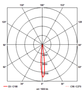
TULI 130 R - 20°
