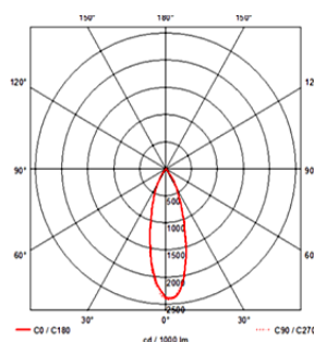
TULI 130 R - 38°
