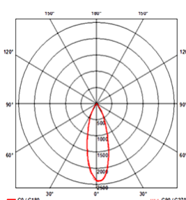
ETOSHA 170 R 38°
