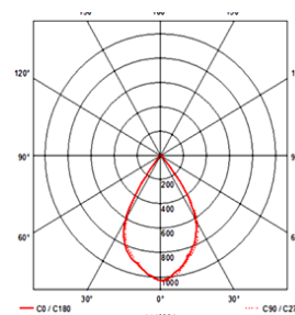
ETOSHA 170 R 60°
