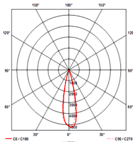
ETOSHA 315X160 L 24°
