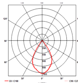
ETOSHA 315X160 L 60°
