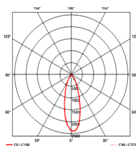
ETOSHA 315X160 L 33°
