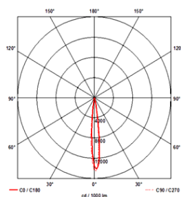
ETOSHA 315X160 L 12°
